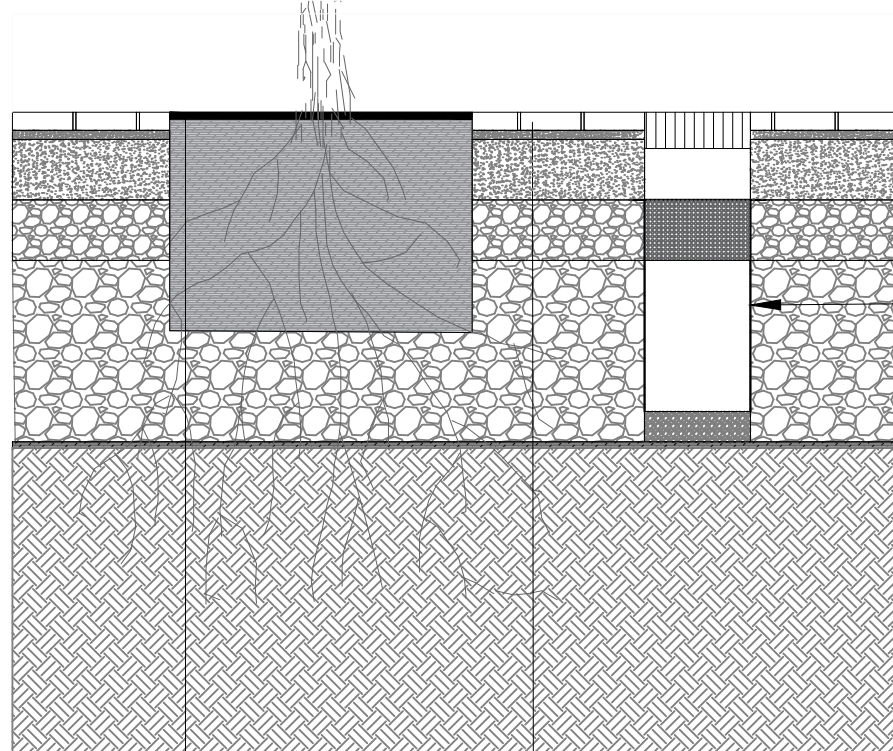
FAHELY VÍZÁTERESZTŐ BURKOLATTAL ÉS LEVEGŐZTETŐ SZEKRÉNNYEL
